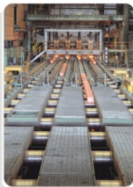
大鋼胚連鑄機
