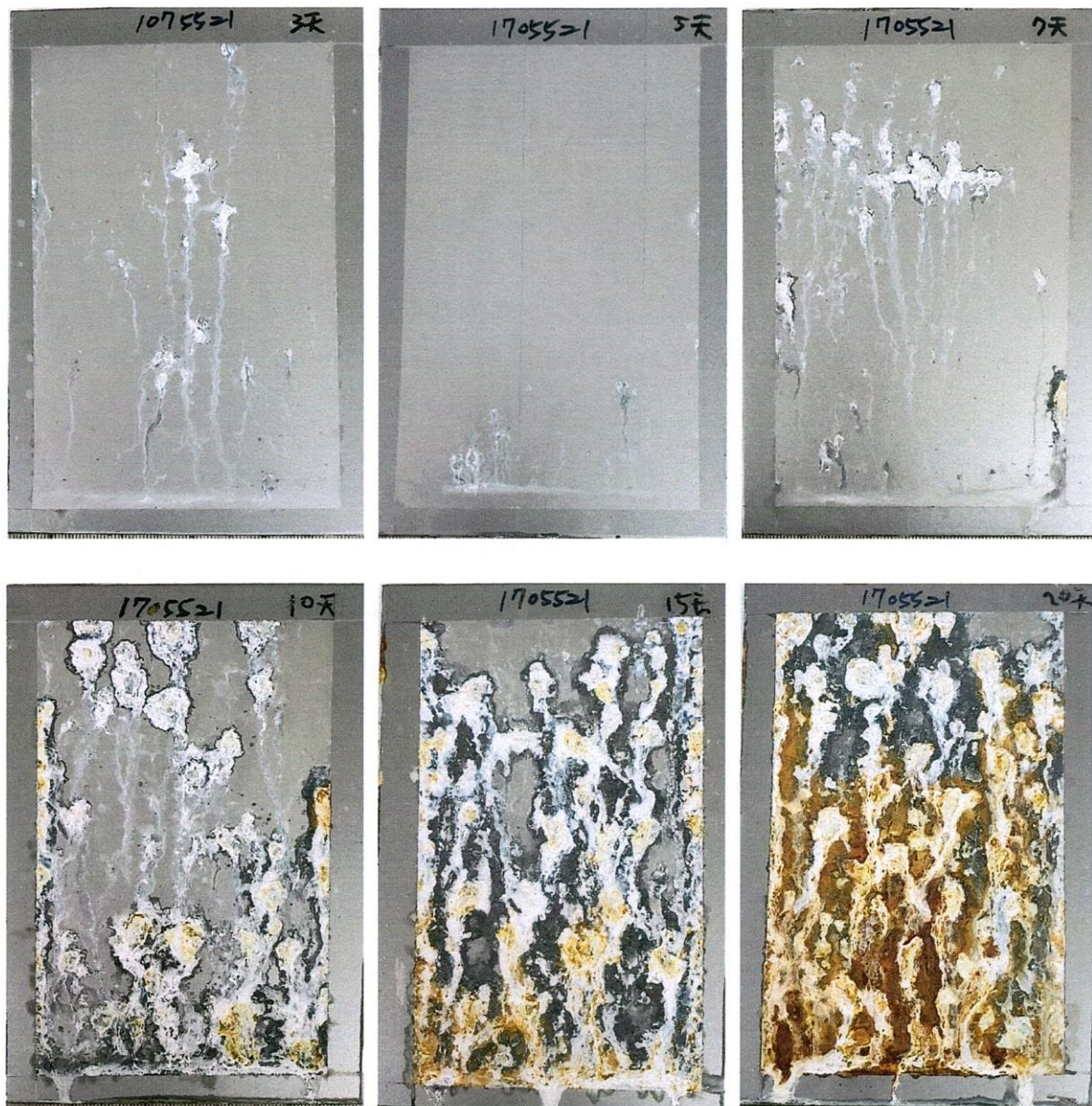
圖 1 1705521(C2 鉻酸處理)鹽霧試驗後外觀
