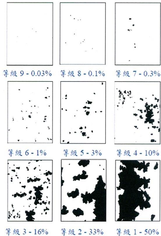
ASTM D610 表面銹蝕等級圖示
