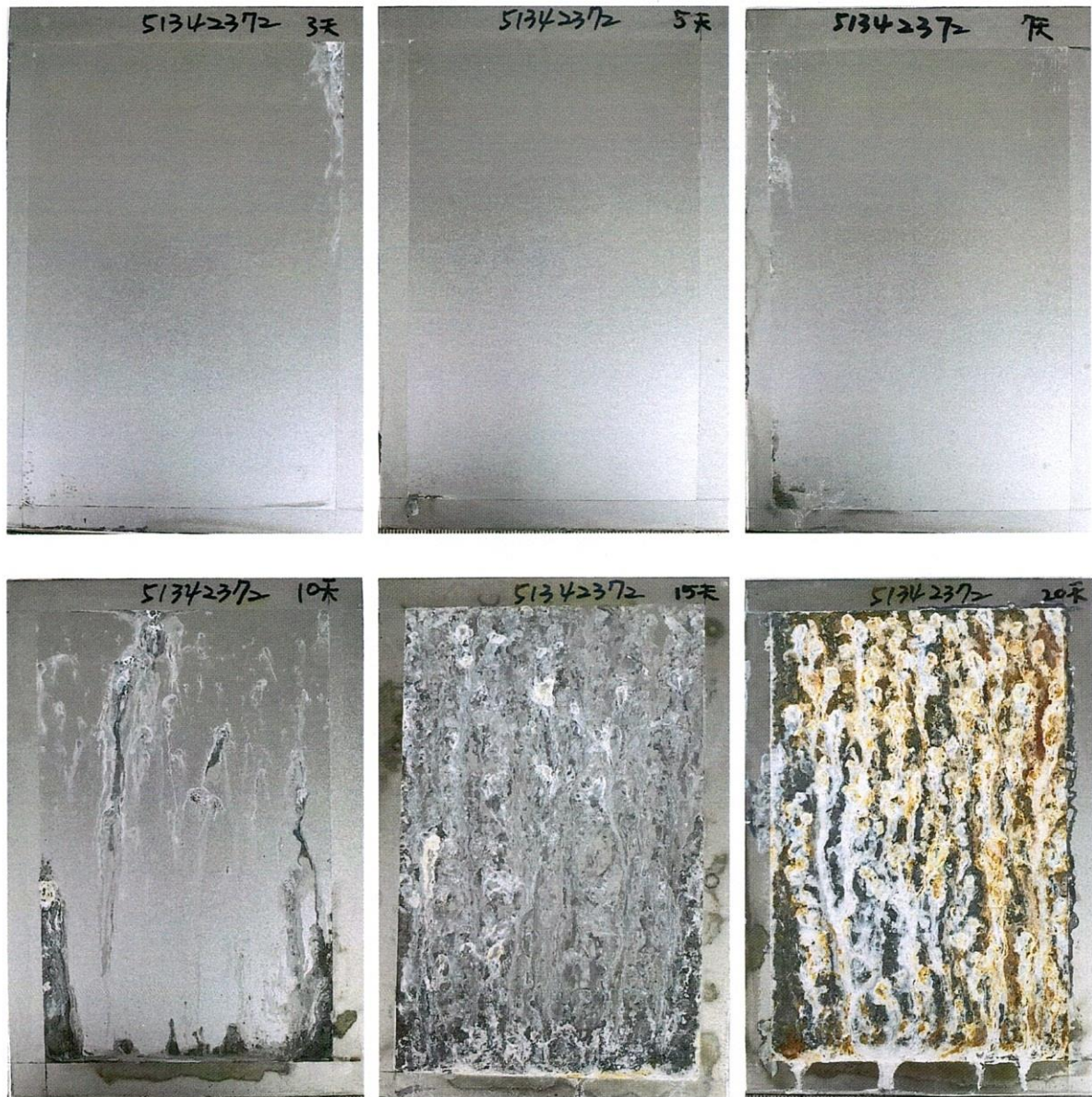
圖 2 51342372(G6 無銘處理)試驗後外觀
