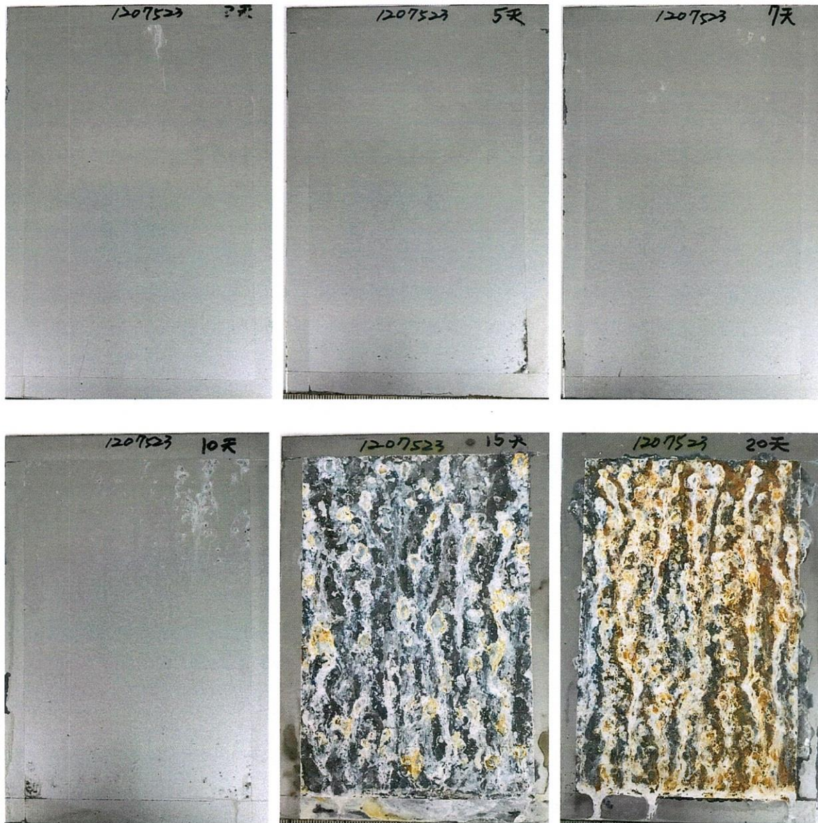
圖 2 1207523(G6 無鉻處理)試驗後外觀
