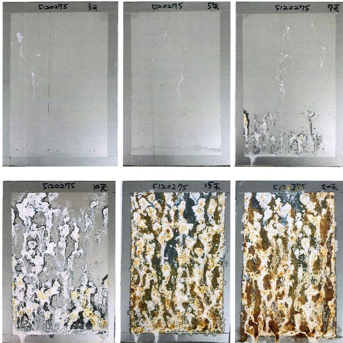
圖 1 5120275(C2 鉻酸處理)鹽霧試驗後外觀
