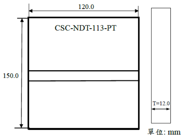
圖二 CSC-NDT-113-PT 試片示意圖
