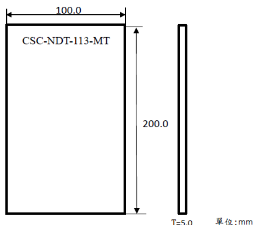
圖一 CSC-NDT-113-MT 試片示意圖
